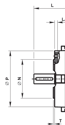
Kołnierz B14
