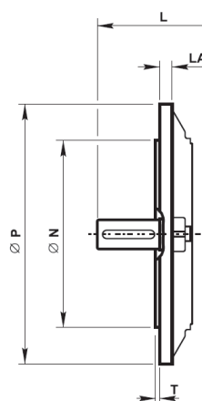
Kołnierz B5
